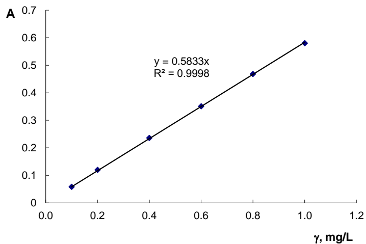
3.1. att. Kalibrēšanas taisne Fe(II) jonu fotometriskai noteikšanai ar 1,10-fenantrolīnu ( \lambda = 510 \text{ nm} , b = 3 \text{ cm} )
